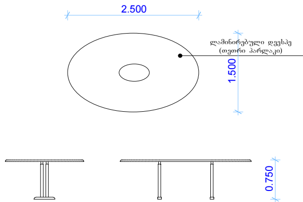
ავეჯის ელემენტი №21 საკონფერენციო მაგიდა
