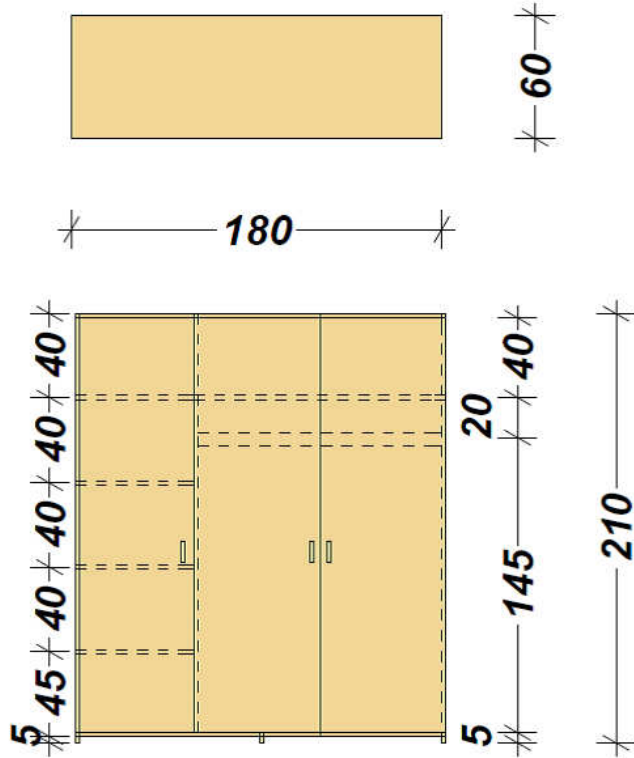
ავეჯის ელემენტი №22 ტანსაცმლის კარადა ჩვეულებრივი კარით
