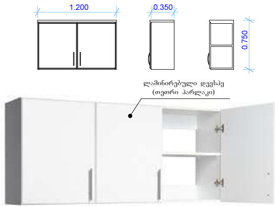
ავეჯის ელემენტი №20 კედელზე ჩამოსაკიდი კარადა
